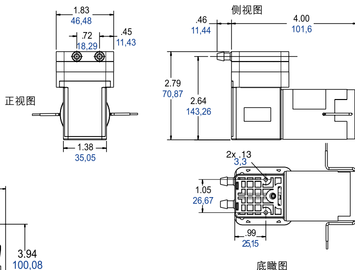
DC直流电型号 英寸/mm
