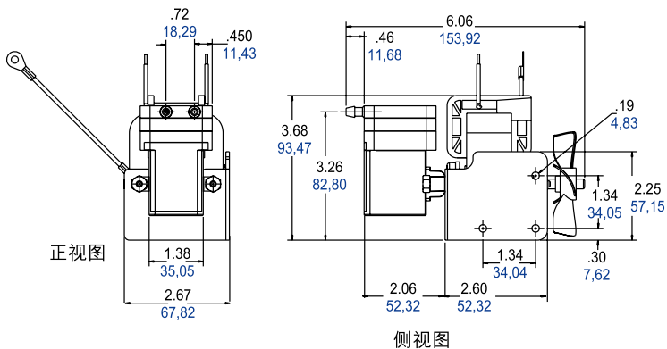
AC交流电型号 图解A (侧面固定底座托架) 英寸/mm
