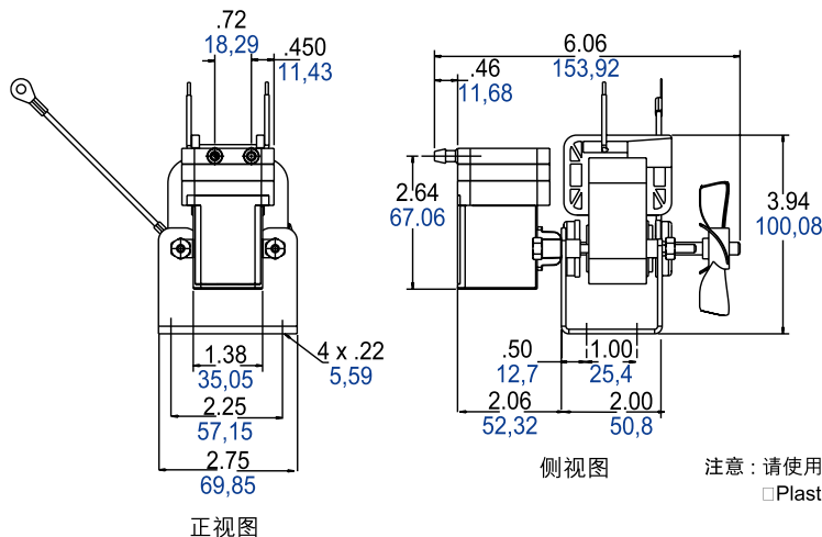
AC交流电型号 图解B (U型底座托架) 英寸/mm
